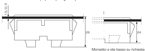
Dimensioni Esterne Display D64 (7 segmenti)
