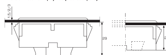
Dimensioni Esterne Display D63 (matrice di punti)
