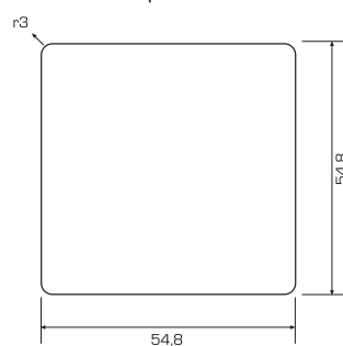
dimensione foro su piastra
